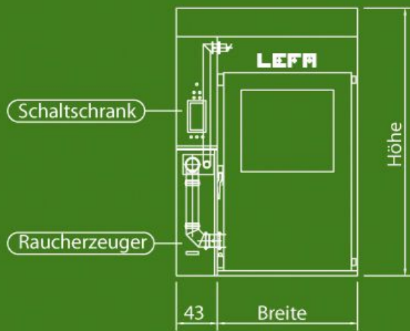
Frontansicht
